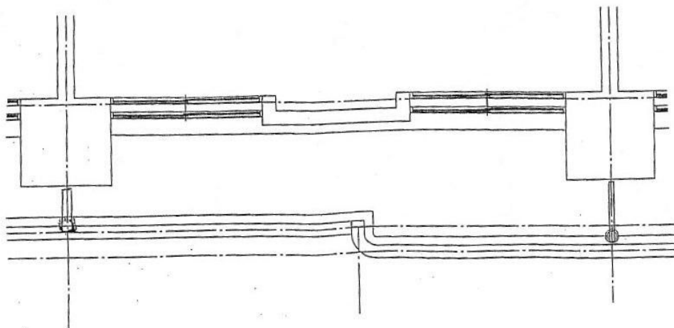
平面図(不具合箇所の記入をお願いします)
